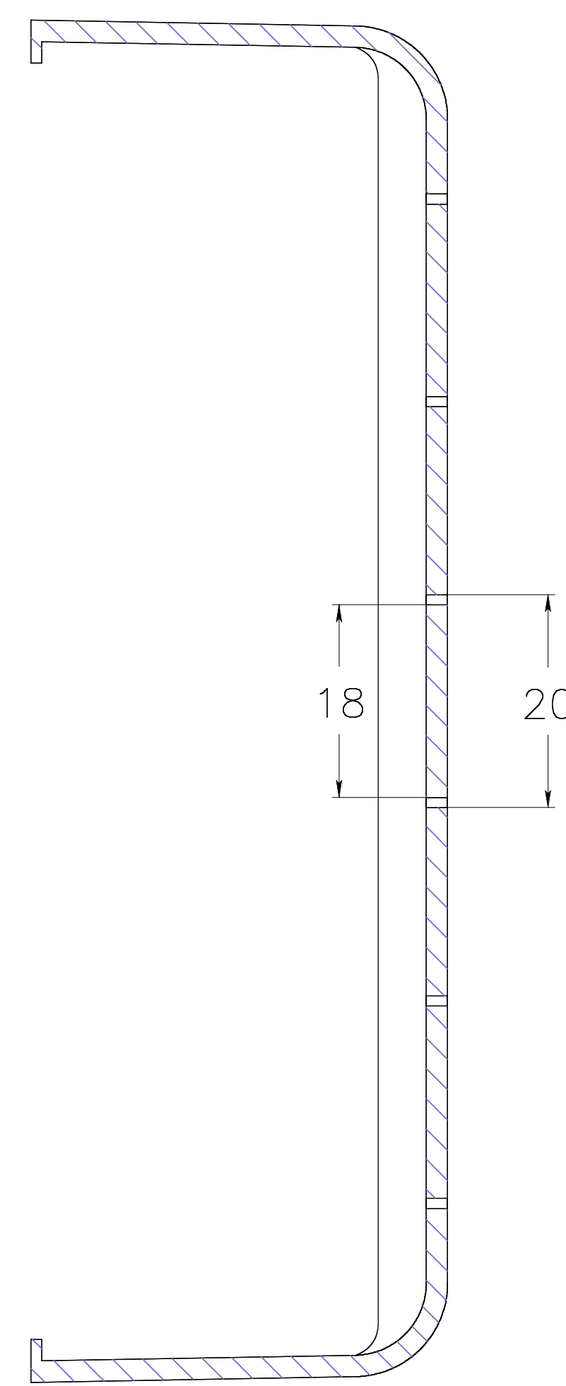
section DD
