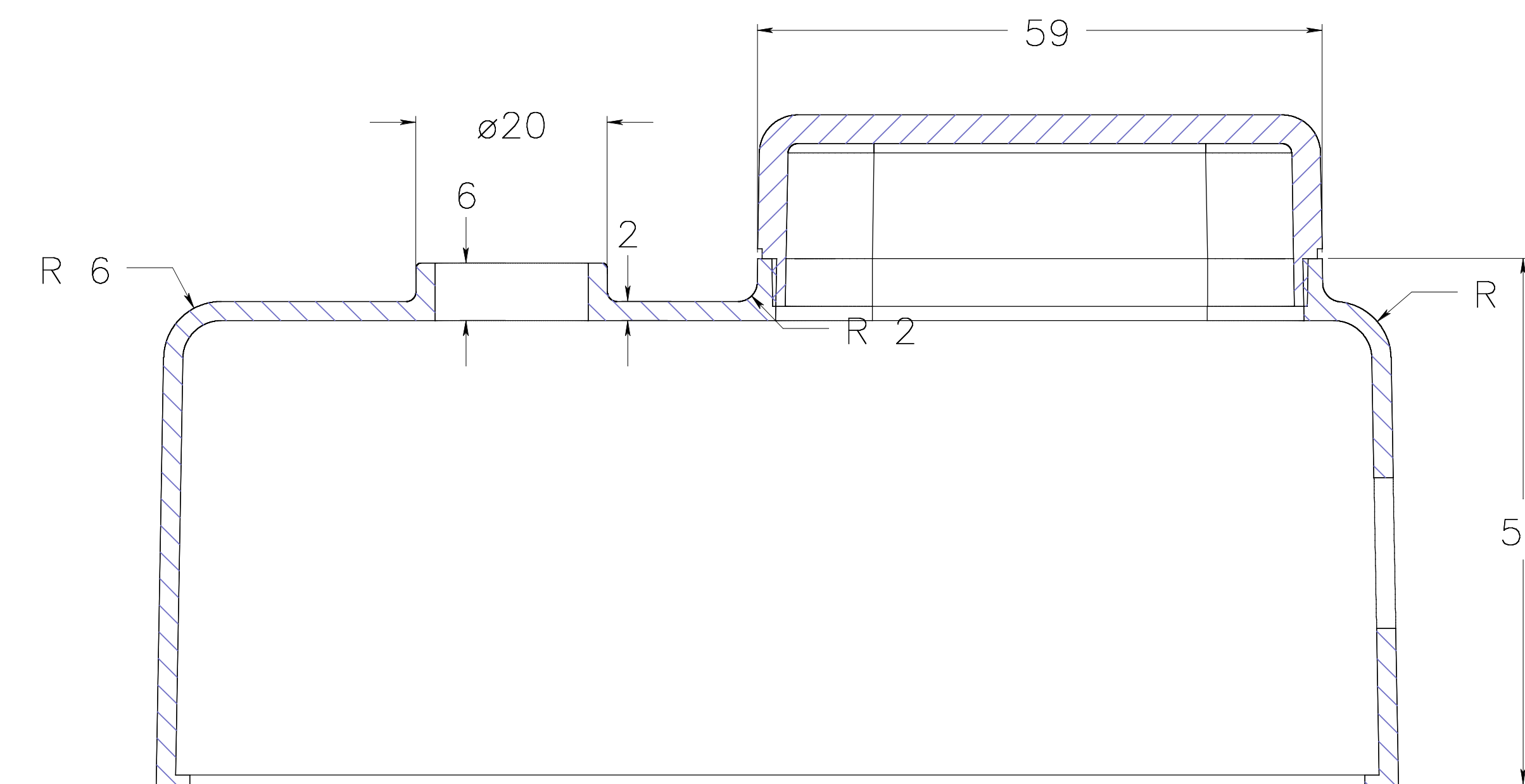
section DD
